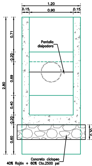
CORTE B-B' CANAL DISIPADOR ESC 1:25
