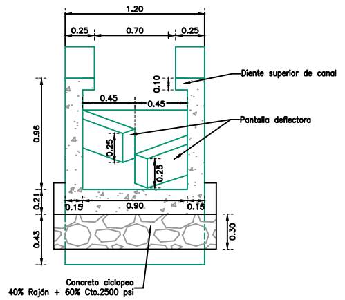
CORTE C-C' CANAL DISIPADOR ESC 1:25
