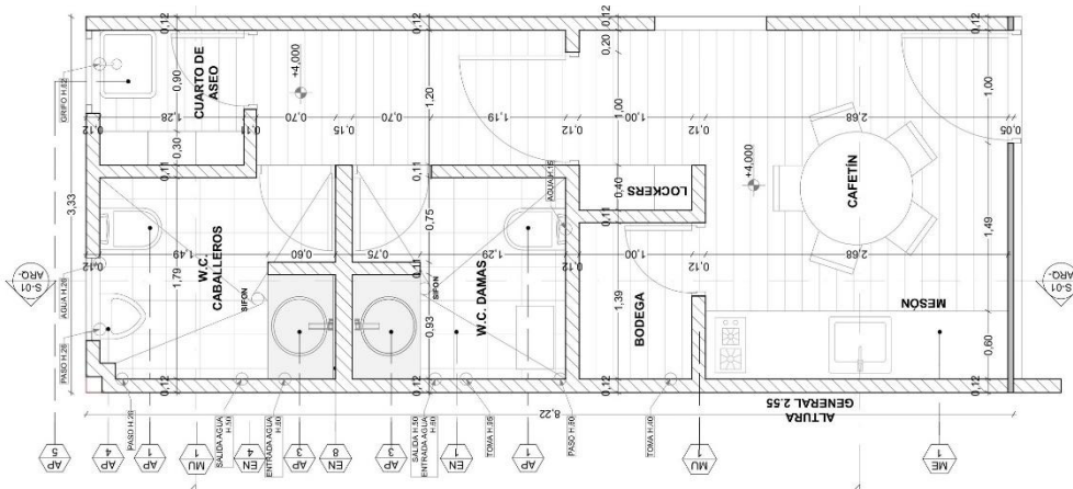
PLANTA PROPUESTA DISEÑO ESC 1:25
